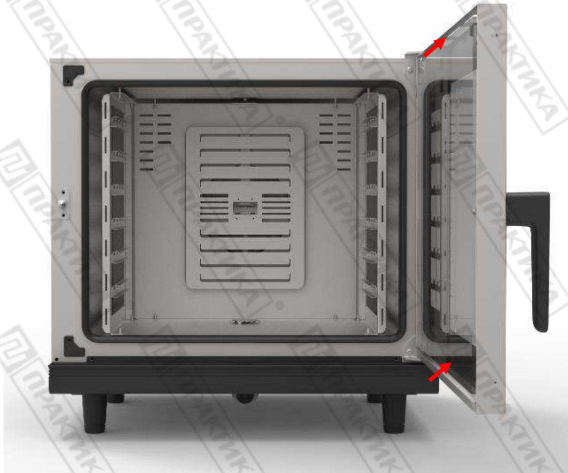
Рисунок 45. Стекланный зажим
